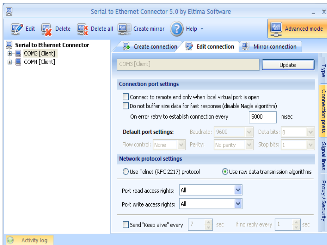
Рис.2. Пример настройки виртуального последовательного порта com3 (вкладка Connection prefs).
